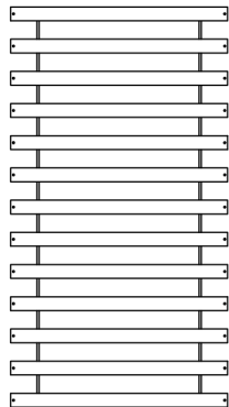
B Upper Bed Slats x 1
