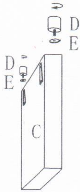
A*1
